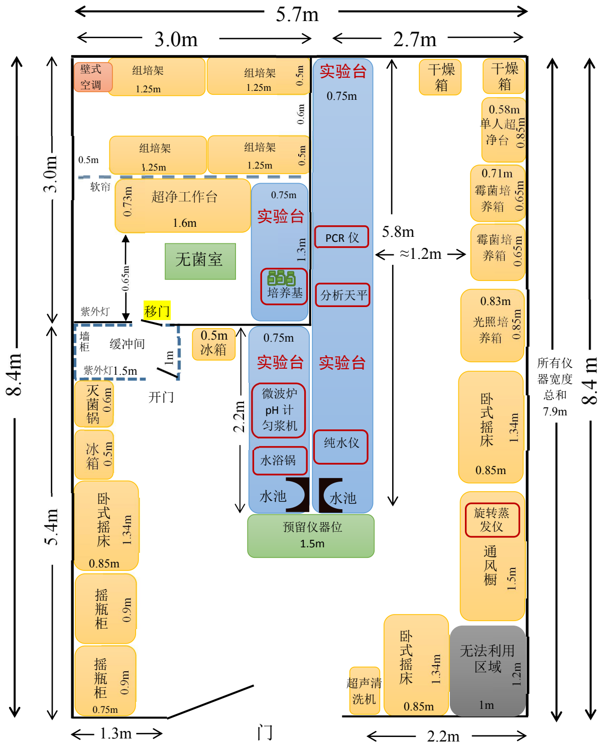
内生真菌实验室设计草图 (20170718)
